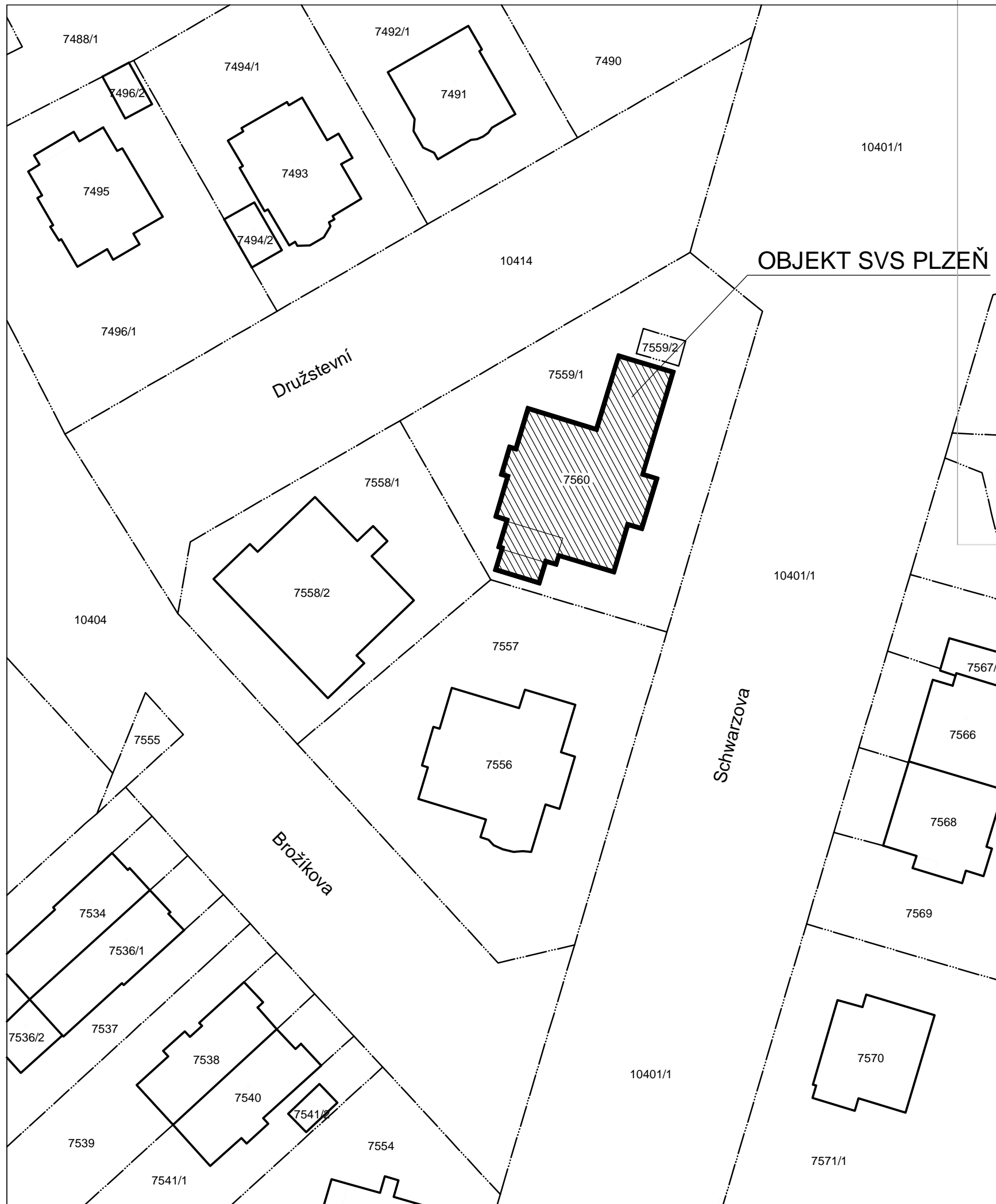
Situační výkres širších vztahů
